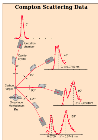
Figur 2.13: Skisse av eksperiment som demonstrerer Compton-effekten, og data fra Comptons opprinnelige eksperiment, som viser opptelling av antall fotoner som funksjon av fotonets bølgelengde. Fotonene kommer oppover fra røntgenrøret, og apparaturen til Compton målte bølgelengdespekter ved forskjellige spredningsvinkler av fotonene (fra http://hyperphysics.phy-astr.gsu.edu , 3/2-2022)
