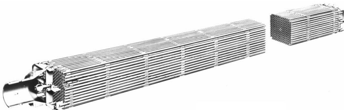
Figur 9.21: Brenselement i trykkvannsreaktor (PWR) Dette element var del av reaktorsystemet til laste- og passasjerskipet NS Savannah. Den sylinderrformede reaktoren hadde en total høyde på ca 15 meter, og en diameter på omtrent 4 meter. Effekten var 74 MW. Designed and built by the Babcock & Wilcox Company. (Fra Wikipedia)
