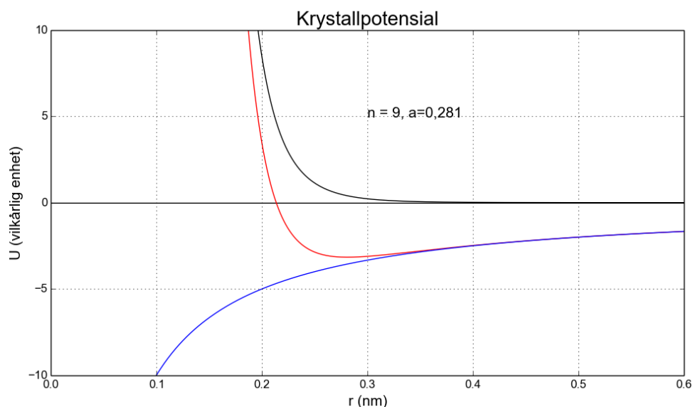
Figur 8.8: NaCl krystall U(r) med n=9 og r_0 = a = 0,281 nm
