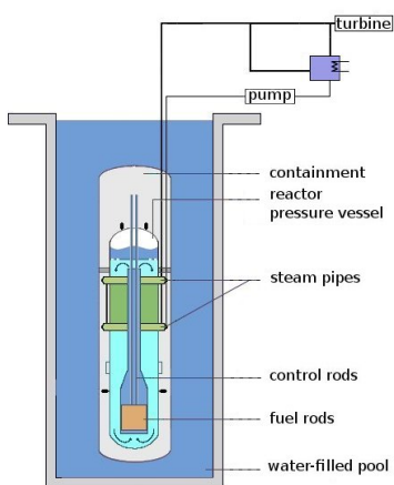
Figur 9.23: Skjematisk oppbygging av en lettvannsreaktor. Wikipedia, [49]
