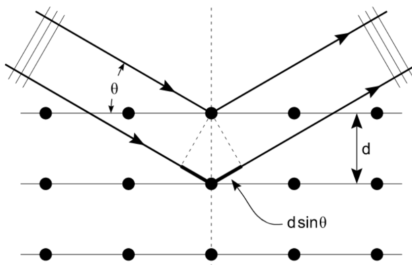
Figur 8.1: Bragg-spredning av kortbølget lys på krystaller. Lys reflektert fra forskjellige atomære lag gir konstruktiv interferens ved vinkler som avhenger av gitteravstanden. Fra Wikipedia [39].
