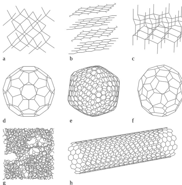
Figur 8.5: Åtte allotroper av karbon: a) Diamant; b) Grafitt; c) Lonsdaleitt; d-f) Fullerenener; g) Amorft karbon; h) Karbon nanorør. Fra Wikipedia [40]
