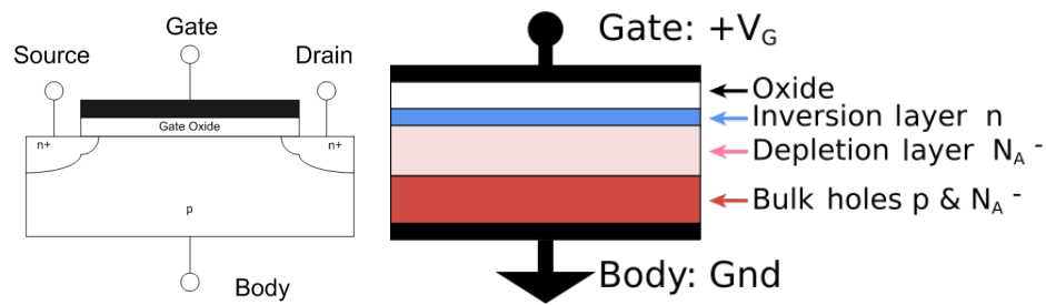
Figur 8.24: Felt-effekt transistor. Til venstre er det ingen påtrykt spenning. Til høyre er det satt positiv spenning på 'gate'. Da skyves huller mot terminalen nederst, og det lages en deplesjonssone uten frie ladninger. Men de n-dopede områdene under 'Source' og 'Drain' øker i utstrekning, og når V_G er høy nok er det dannet en ledende kanal mellom de to terminalene. Tykkelsen av kanalen, og dermed strømmen mellom 'Source' og 'Drain' kontrolleres av V_G . (fra Wikipedia [45])
