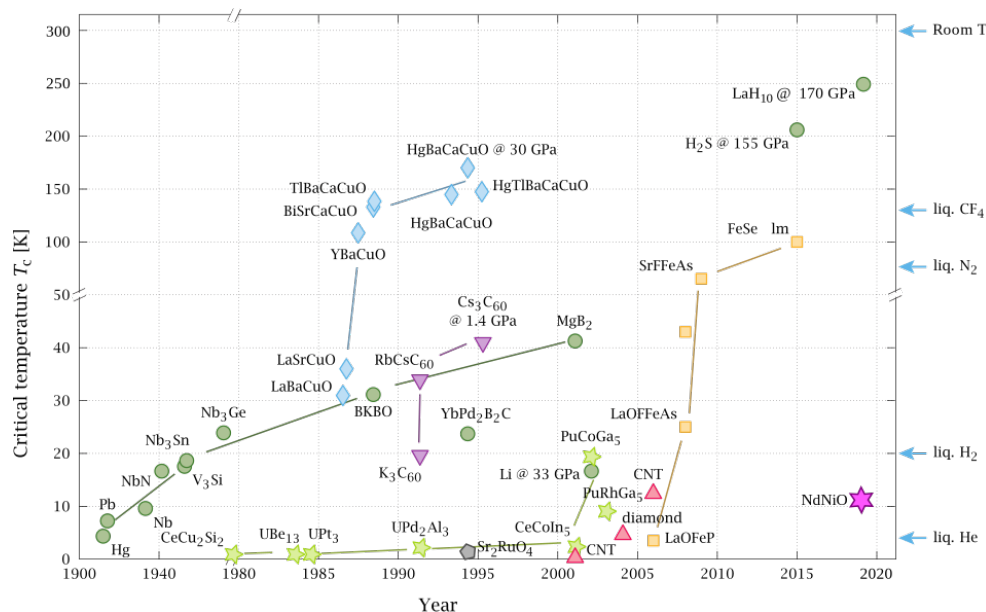
Figur 8.27: Utvikling av kritisk temperatur for superledende materialer. Fra Wikipedia [47]
