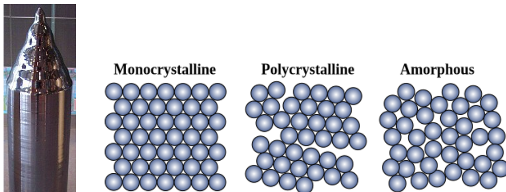
Figur 8.19: Venstre: En stav bestående av en monokrystall av silisium. Slike staver lages med forskjellige diametre, f.eks 150 mm og 300 mm. Staven sages i tynne skiver, typisk 0,3mm. Så prosseseres skivene. De dopes med Bor eller Fosfor for å lage p- eller n- type skiver. Prosessen videre avhenger av hva skivene skal brukes til. Høyre: Forskjellige former av silisium Fra Wikipedia [43].
