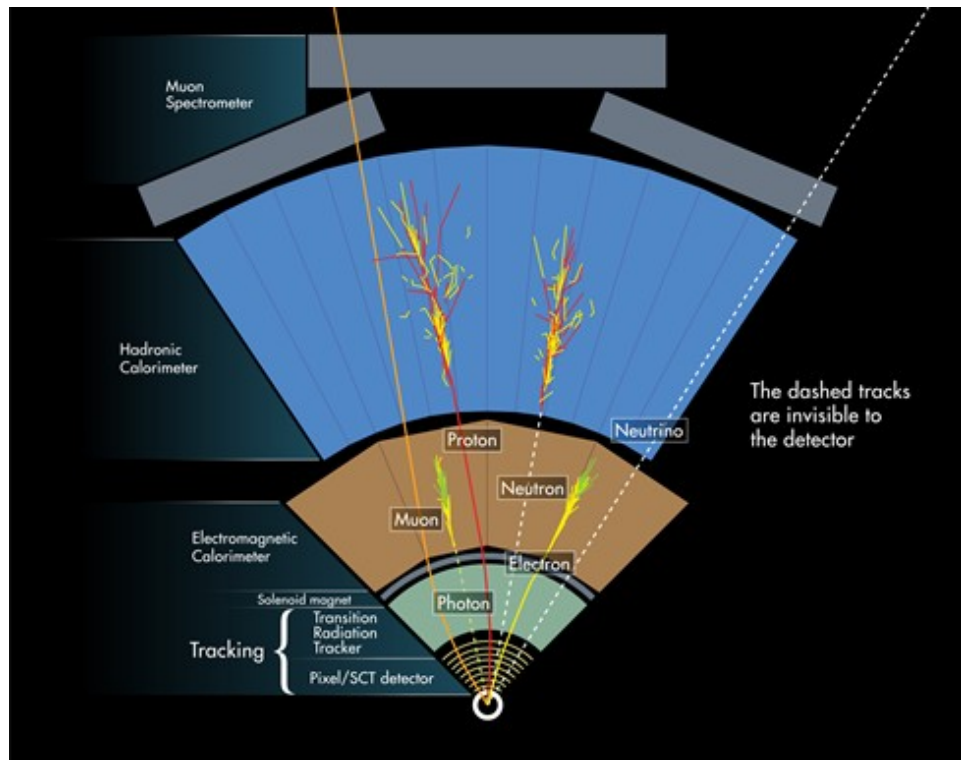
Figur D.2: Prinsippskisse for ATLAS detektoren (fra CERN). Det er to typer spordetektorer. Her måles bevegelsesmengden til alle ladde partikler. Fotoner og elektroner vil stoppe helt i det elektromagnetiske kalorimeteret. Protoner og pioner vil fortsette, og avgi all energi i Hadronkalorimeteret. Myoner vil traversere helt ut til myonspektrometeret. De nøytrale nøytrinoene vil ikke vekselvirke i det hele tatt, og forsvinne ut av detektorsystemet. Men ved å se på energibalansen i systemet har man mulighet til å finne ut hvor mye energi som har forsvunnet uten å vekselvirke. I tillegg til nøytrinoer kan ubalanse i energiregnskapet være en signatur for mystiske partikler som ikke er del av vår standardmodell.
