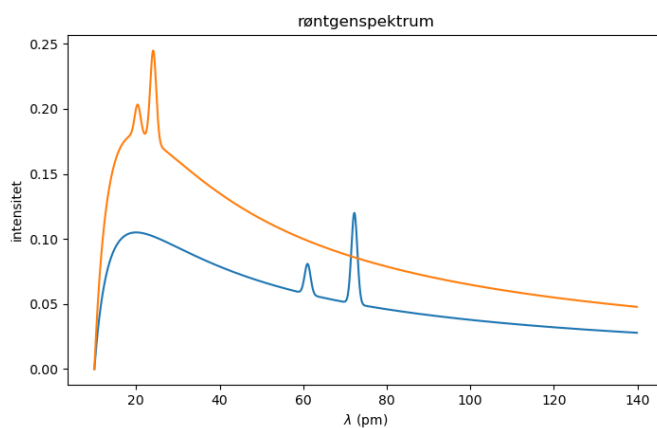
Figur 2.10: Intensitetsfordelinger, (spektre) fra røntgenstråling, skjematisk for Molybden ( Z=42 ) og Wolfram ( Z=72 ) ut fra formlene 2.9 og 2.12. Høyden og bredden av de skarpe toppene vil avhenge av oppløsningsevnen til registreringssystemet.
