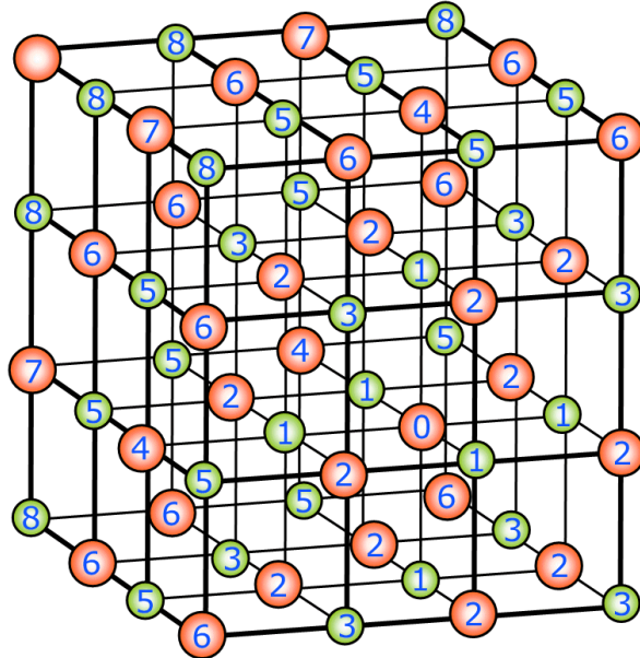
Figur 8.6: NaCl krystall (fra Wikipedia [41]).
