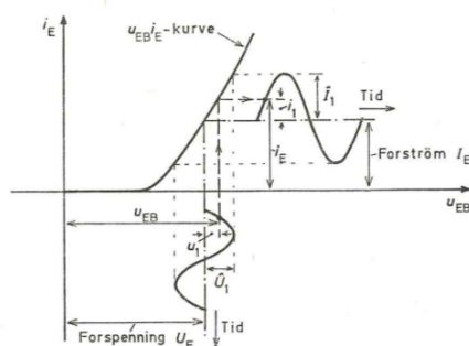
Fig. 4.9. Når inngangskretsen tilføres en vekselspenning med amplitudeverdi \hat{U}_1 i serie med forspenningen U_E , vil emitter-basisspenningen u_{EB} svinge periodisk mellom U_E + \hat{U}_1 og U_E - \hat{U}_1 , så emitterforstrømmen I_E får en overlagret vekselstrømskomponent med amplitudeverdi \hat{I}_1 .
