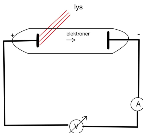
Figur 2.3: Skjematisk tegning av apparatur til å måle stoppepotensialet til elektroner som frigjøres når lys treffer et materiale (en fotokatode). Lyset forårsaker en strøm av elektroner mot den negative terminalen. Det går strøm så lenge det fins elektroner med nok energi til å nå fram til anoden (som i dette eksperimentet er lagt på et negativt potensial). Man justerer spennin-gen inntil det slutter å gå strøm. Denne spenningen gir da den maksimale elektronenergien (i elektronvolt)
