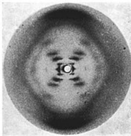
Figur 8.3: Diffraksjonsbilde 'Photo 51' tatt under studium av DNA-molekylet av Rosalind Franklin og Ray Gosling.
