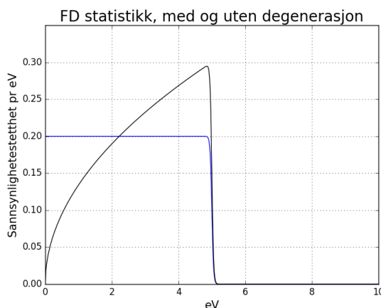
Figur 7.8: Fermifordelingen, og Fermi-Diracfordelingen multiplisert med degenerasjonsfaktoren (lign. 7.68), normerte, når det antas at temperaturen (mer presist: kT ), er mye lavere enn Fermienergien.
