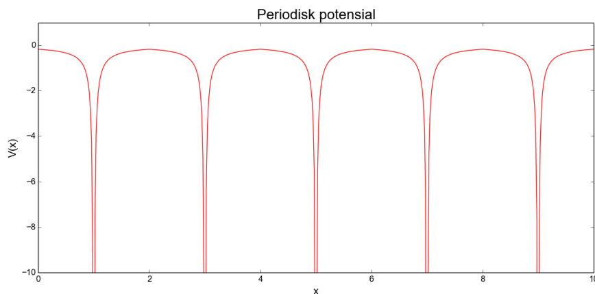
Figur 8.11: Coulomb-potensialet fra en rekke positive ladninger.
