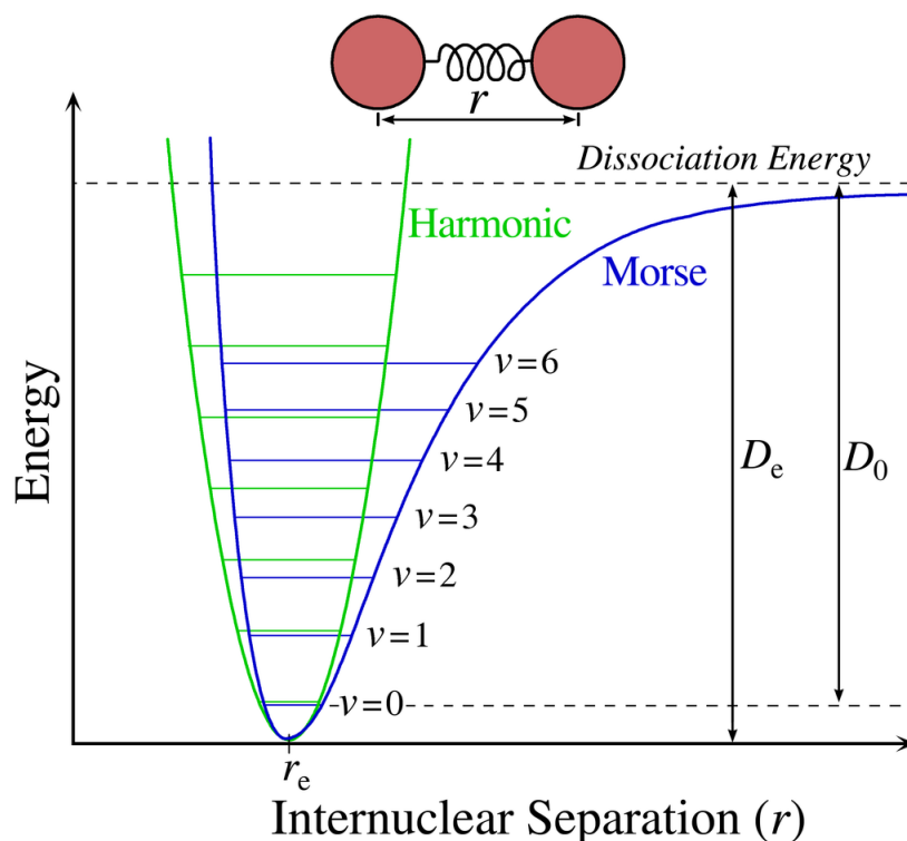
Figur 6.2: Sammenligning av Morse-potensial og harmonisk oscillator. Fra Wikipedia [35]
