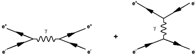
Figur 10.3: Feynman-diagram som bidrar til elastisk spredning mellom et elektron og et positron. a) Annihilasjon b) Fotonutveksling. For å finne virkningstverrsnitt for reaksjonen må man addere amplitudene og kvadrere resultatet.
