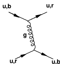
Figur 10.13: Feynman-diagram av kollisjon av to u-kvarker, med gluonutveksling. Kvarken har fargeladning som overføres med gluonet til den andre kvarken. Verteks-faktoren her er kvadratroten av den sterke koblingskonstanten, \alpha_s
