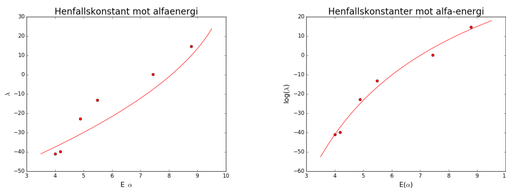
Figur 9.10: logaritmen til henfallskonstanter mot alfaenergi (i MeV) for to modeller av potensialet. De røde linjene er modellene. Til venstre barriere som firkantet boks. Til høyre har vi Gamows modell, med frastøtning på grunn av Coulombpotensialet. Vi ser at denne modellen passer godt med datapunktene.
