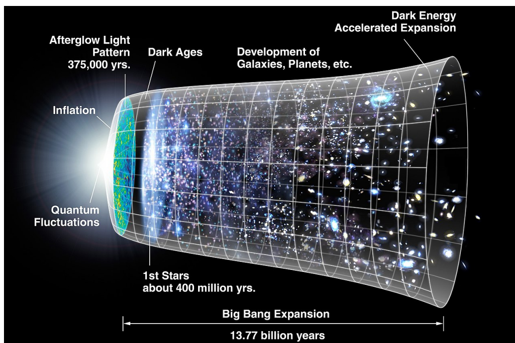
Figur 11.4: Universets utvikling. Fra Wikipedia (NASA/WMAP Science Team - Original version: NASA; modified by Cherkash). Det er klistret inn et 'bilde' av dagens temperatur på den kosmiske bakgrunnstrålingen, til venstre på tidsaksen. Det var da universet var strålingsdominert, og strålingen ble 'fri', med liten vekselvirkning med materien forøvrig. Satellitteksperimentet WMAP har produsert dette kartet over strålingstemperaturer. Planck-satellitten har laget et enda mer detaljert kart.
