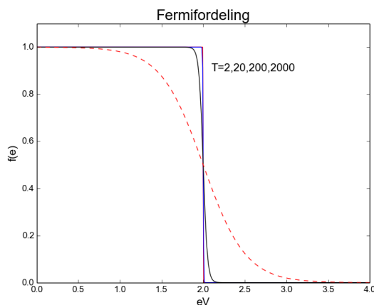
Figur 7.7: Fermi-Dirac-fordelingen for forskjellige temperaturer. I figuren er \mu satt lik 2 elektronvolt.
