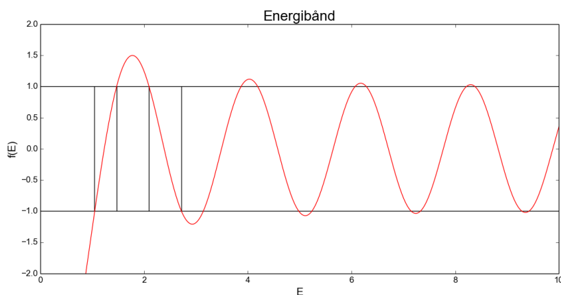
Figur 8.12: Løsninger av S.L. må ha energier som er i områdene der den røde kurven, f(E) ligger mellom -1 og 1.
