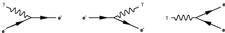
Figur 10.1: Feynman-diagram a) Fotoabsorpsjon, b) Bremsstråling, c) Parproduksjon. Tiden løper fra venstre mot høyre. Linjene sier ingen ting om bevegelsesmengder og retninger, men bevaring av energi og bevegelsesmengde må være oppfylt. Vi skal se at dette nødvendiggjør konseptet med virtuelle partikler
