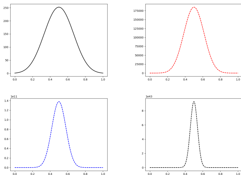
Figur 7.3: Fordeling av antall måter man får utfall 'kron' på, når man har kastet h.h.v. 10, 20, 40 og 150 mynter. Antallene er plottet som funksjon av andel 'kron'. Legg merke til at fordelingen blir smalere etterhvert som N øker. Legg også merke til hvor stor funksjonsverdien \Omega(n_k) = N/2 blir for store N . Når du gjør 150 kron/mynt kast, så kan man få 75 'kron' og 75 'mynt' på omtrent 9 \times 10^{43} måter!
