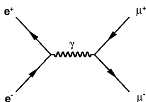
Figur 10.4: Feynman-diagram for produksjon av et par myoner gjennom elektron-positron annihilasjon. Alle fermioner, forutsatt at de har elektrisk ladning, kan produseres i par på denne måten, bare det er nok energi i annihilasjonen.
