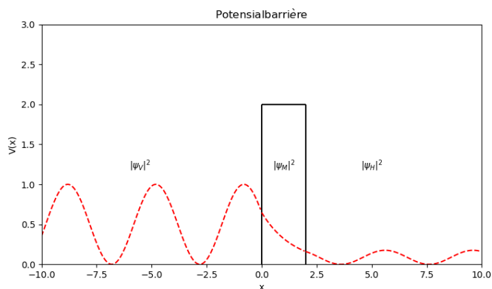
Figur 3.6: Sannsynlighetstetthet for en strøm av partikler som kommer mot høyre og treffer en potensialbarriere, som et øyeblikksbilde med en statisk bølgefunksjon
