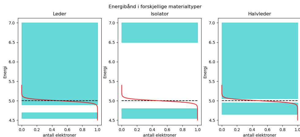
Figur 8.13: Forhold mellom fermienergi og båndgap i faste stoffer. Fermi-Diracfordelingen er tegnet inn med E_F = 5\text{eV} og en temperatur på 300K, og angir en kurve proporsjonal med 'teoretisk' antall elektroner uten degenerasjon (rød linje). De turkise feltene angir lovlig energibånd (valensbånd nederst, ledningsbånd øverst), og de hvite feltene er båndgap, energier som er forbudt for elektronene.
