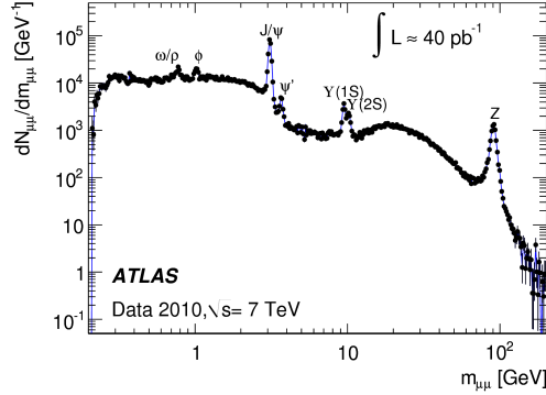
Figur 10.9: Fordeling av invariante masser av \mu^+\mu^- par funnet i data fra ATLAS detektoren. Man ser at det er produsert kortlivede partikler med forskjellige masser, som har henfalt til \mu^+\mu^- par. Legg merke til at den vertikale skalaen er logaritmisk
