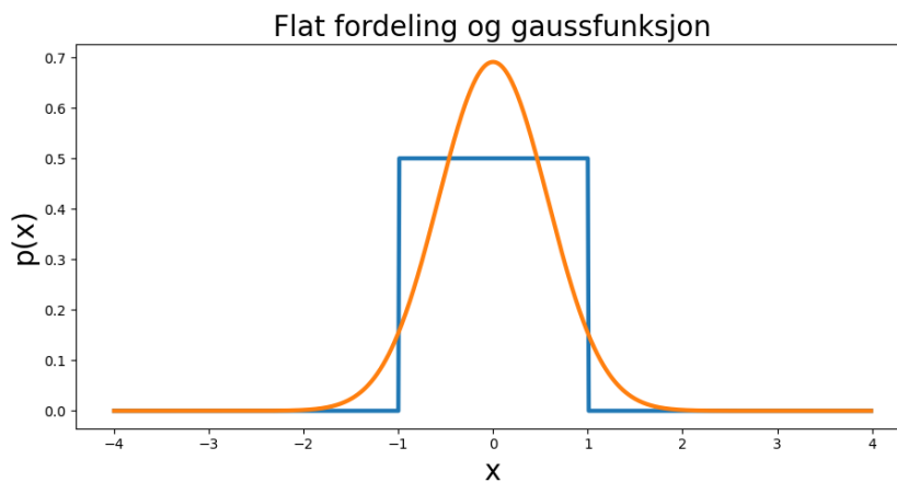
Figur 2.7: Flat sannsynlighetsfordeling, og gaussisk sannsynlighetsfordeling med samme standardavvik (i denne figuren lik 2/\sqrt{12} \approx 0,58 ). Begge fordelingene har samme normalisering (samme verdi av \int_{-\infty}^{\infty} p(x)dx ).
