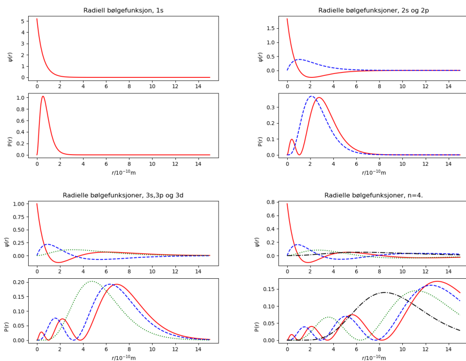
Figur 4.4: Radialfunksjoner og sannsynlighetsfordelinger i r for n = l, 2, 3, 4 og l < n (x-akse i Ångström). Heltrukne røde linjer er for l = 0 . Disse har verdier forskjellig fra null i r = 0 . Men sannsynligheten for at elektronet skal befinne seg i r = 0 er likevel 0 fordi volumelementet går mot null. Stiplet blå linje er for l = 1 , prikket grønn for l = 2 og prikk-strek er for l = 3
