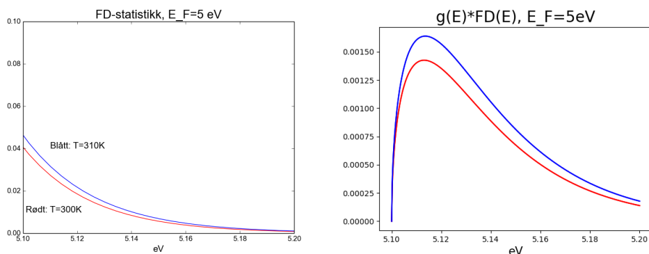
Figur 8.14: Fermi-Dirac fordeling når Fermienergien er 5 eV (venstre). For- deling modulert med faktor g(E) = \sqrt{E - 5.1} (høyre)
