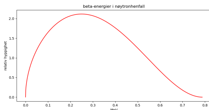
Figur 9.11: Spektrum av betaenergier fra nøytronhenfall, slik det framkommer i grove trekk. (Se f.eks. [19]) Her vises elektronets kinetiske energi (total energi minus hvileenergien på 511 keV)
