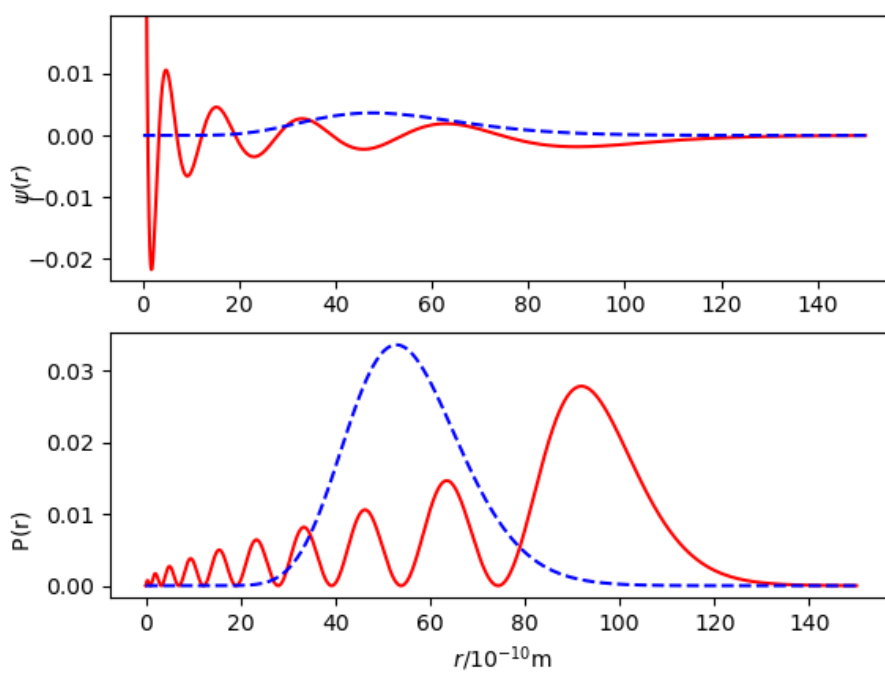
Figur 4.5: En høyt eksitert tilstand. Heltrukken rød linje er for l = 0 . Stiplet linje er for l=9 . Iflg. Bohrmodellen har banen for n = 10 en radius på 10^2 a_0 \approx 53 \times 10^{-10} \text{ m}
