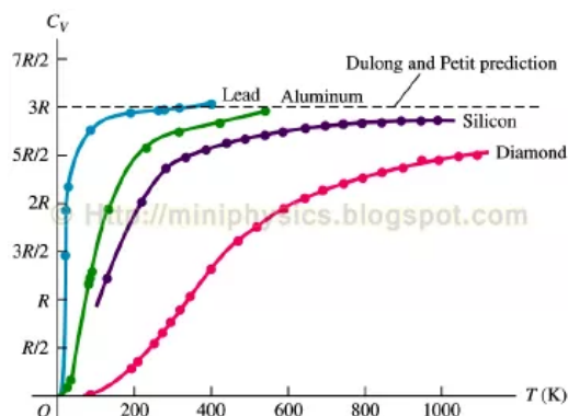
Figur 7.14: Varmekapasitet for forskjellige stoffer som funksjon av temperatur.
