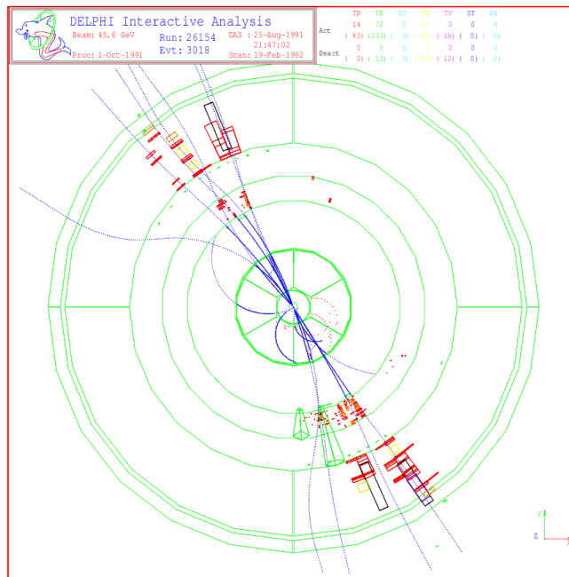
Figur 10.14: Bilde som viser et eksempel på prosessen e^+e^- \rightarrow q\bar{q} i DELPHI eksperimentet ved CERNs LEP (Large Electron Positron Collider). Projeksjon i planet som er vinkelrett på stråleretning, der elektronet og positron har gått hver sin vei og kollidert i sentrum av bildet. Et kvark-antikvark par er dannet gjennom annihilasjon (se fig. 10.4 med kommentar). Kvarkene har umiddelbart dannet hadroner, (flest mesoner slik som \pi -mesonet) i to kollimerte bunter ('jeter'), som vi ser sporene av i detektoren.
