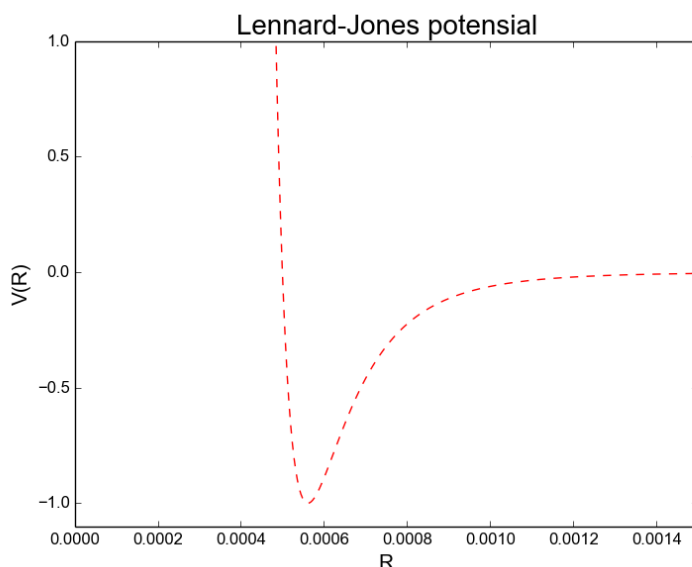
Figur 8.9: Lennard-Jones potensialet mellom polariserte molekyler.
