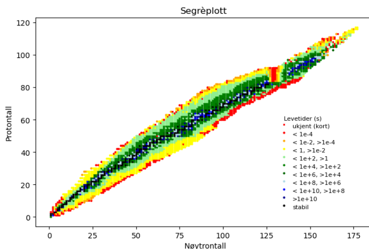
Figur 9.5: Protontall mot nøytrontall for kjente kjerner. Fargekoden viser levetider. Kategorien 'ukjent' er kortlivede nuklider med kun øvre grenser for levetiden. Data fra https://www.nndc.bnl.gov/nudat3 .
