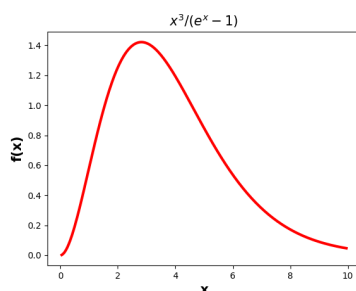
Figur 7.9: Funksjonen x^3/(e^x - 1) .
