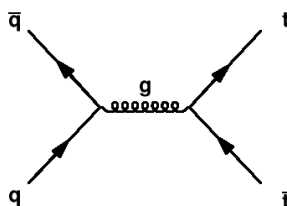
Figur 10.15: Det mest dominerende Feynmandiagrammet for produksjon av topp-kvarken ved Fermilab's Tevatron.
