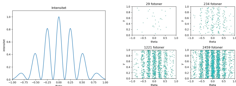
Figur 2.8: Intensitetsfordeling for lys gjennom en dobbeltspalte (til venstre). Til høyre er enkeltfotoner simulert i henhold til intensitetsfordelingen med treffpunkt i en tenkt skjerm. Etterhvert som antall fotoner øker ser man at interferensmønsteret trer fram.
