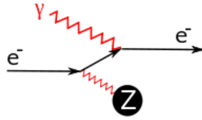
Figur 10.2: Feynmandiagram for fotoelektrisk effekt, slik det må se ut for at alle bevaringslover skal være oppfylt. Den sorte boblen antyder vekselvirkning med en atomkjerne med effektiv ladning Z . Hentet fra tysk Wikipedia den 20/10 2016
