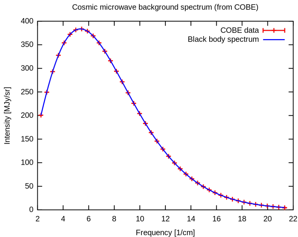
Figur 11.3: Spekter av kosmisk bakgrunnstråling. Formen følger det som forventes utfra Planck's strålingslov med svært god presisjon, og man finner at universets temperatur for tiden er på 2,73 K. Datapunktene vises som røde kryss, men usikkerhetene er for små til at de kan vises i figuren! (Fra Wikipedia: By Quantum Doughnut - Own work, Public Domain, https://commons.wikimedia.org/w/index.php?curid=12958270 )
