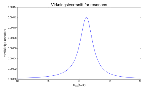
Figur 10.7: Virkningstverrsnitt for en resonans (Breit-Wigner), uten korreksjoner
