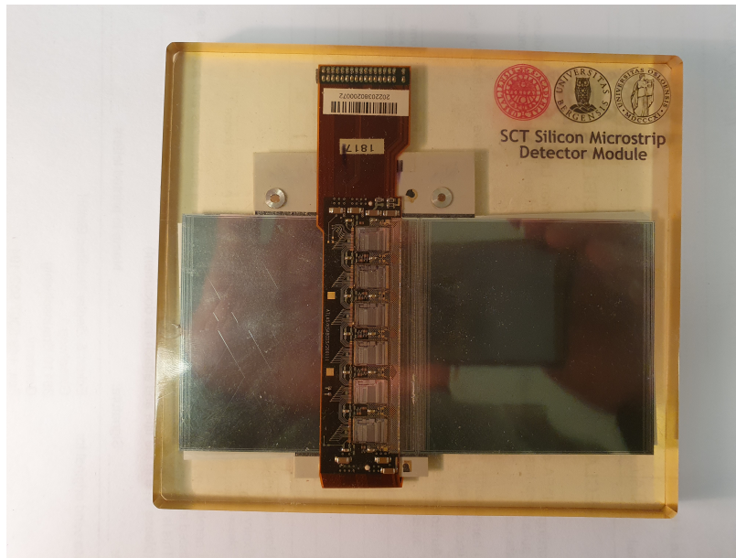
Figur 8.20: En sensormodul bygd opp av fire tynne (ca 280\text{ }\mu\text{m} ) silisiums-sensorer som hver dekker et areal på ca 6\times 6\text{ cm}^2 , og utlesningselektronikk. Sensorene er delt inn i 768 striper. Stripene er koblet sammen parvis, som leses ut individuelt og gir en koordinat som er ca 12 cm lang og 80\text{ }\mu\text{m} bred. Slike moduler var del av ATLAS detektoren ved CERN fra starten og fram til en større oppgradering i 2026-2027, da de blir erstattet med nye moduler som også er laget av silisiumsensorer. (Modul innbakt i plast og stilt ut på forfatterens kontor)
