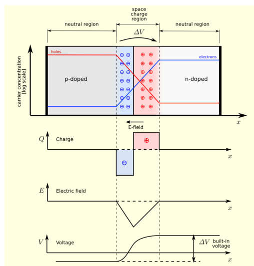
Figur 8.16: En modell for ladningsfordeling, elektrisk felt og potensial i en planar diode. Når man antar uniform ladningsfordeling i områdene med negativ og positiv romladning, vil Poissons ligning gi elektrisk felt og potensial som vist. Figur fra Wikipedia [42].
