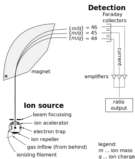
Figur 9.3: Prinsippskisse for massespektrometer, for måling av nuklidemasser, eller identifikasjon av dem. Fra Wikipedia.
