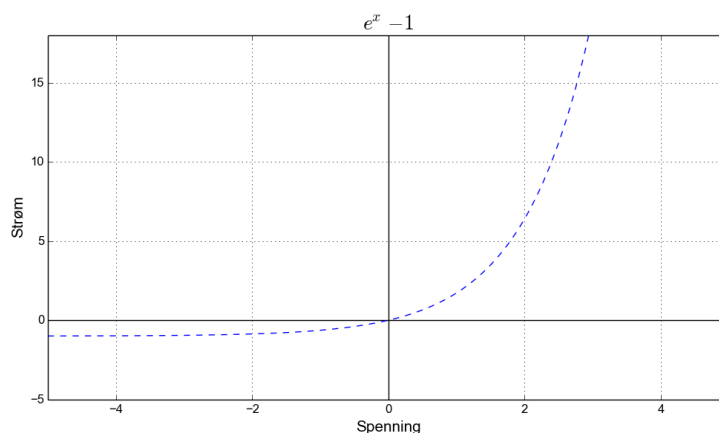
Figur 8.18: Diodeligningen
