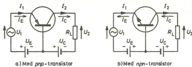
Fig. 4.8. Prinsipp for basiskoplet transistorforsterker.
