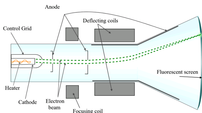
Figur 2.1: Katoderør. Dette bildet viser hvordan elektronene styres mot en skjerm. Styringen kan være hurtig og gjøres med høy presisjon. Fjernsynsapparater, dataskjermer og oscilloskop var bygd opp rundt slike rør fram til slutten av 1990-årene. Fra Wikipedia [32]
