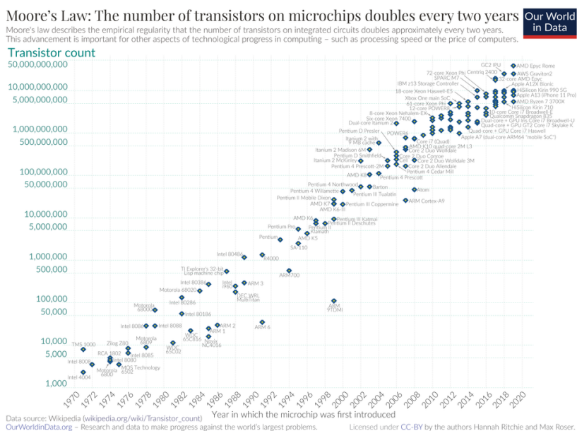
Figur 8.26: Moore's 'lov' som viser at antall transistorer som kan integreres på en mikrochip har doblet seg annethvert år siden 1970. Fra Wikipedia [46].
