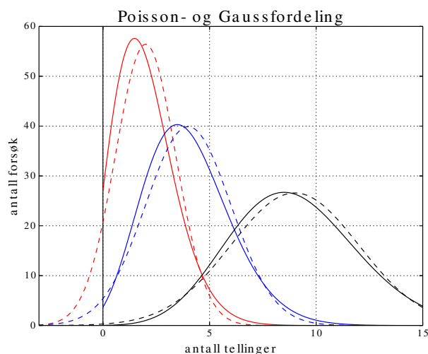
Figur B.2: Poissonfordeling (heltrukken) og Gausstilmærming (stiplet) for 200 forsøk med middelværdier h.h.v 2, 4 og 9. Poissonsannsynlighet er bare definert for hele tall, men er her likevel tegnet som kontinuerlig funksjon (se tekst)
