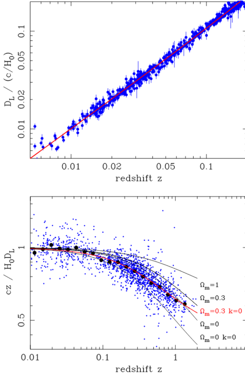
Figur 11.2: Avstand som funksjon av rødsift for supernovaer (fra [31]). I det nederste plottet er avstanden dividert med den lineære trenden gitt av Hubble's lov. Da vises hvordan sammenhengen ikke lenger er lineær ved høye rødsift. I \Lambda -CDM modellen kan man forutsi hvordan denne sammenhengen må være for gitt innhold i universet. De svarte punktene viser median av observasjonene for forskjellige rødsift, og linjene viser forutsigelser av trenden for forskjellige materieandeler og geometrier av universet
