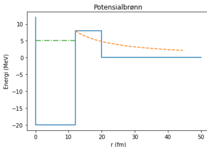
Figur 9.9: To modeller for potensialbrønn: Barriere er enten en firkantet boks eller et Coulombpotensial. Energinivået til en alfapartikkel er antydnet, og sannsynlighet for tunnelering er sterkt avhengig av dette energinivået.
