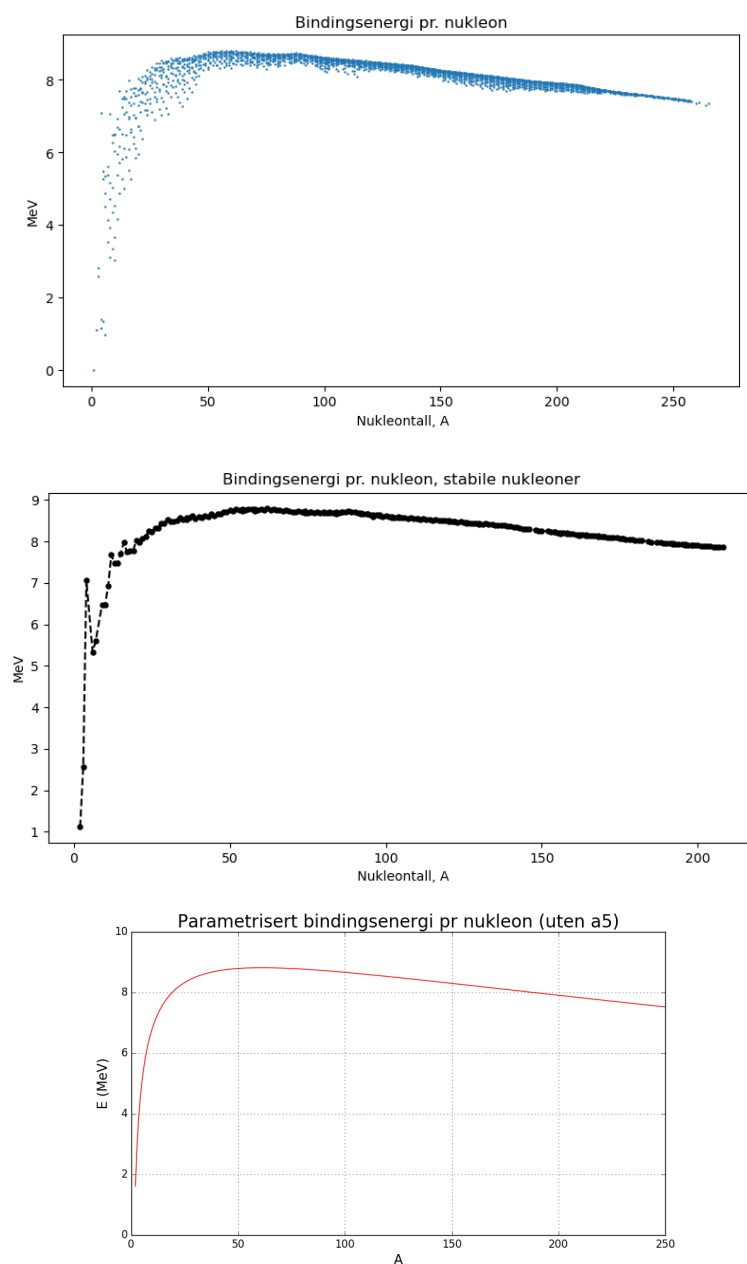
Figur 9.4: Bindingsenergi per nukleon som funksjon av massetallet, A . Det midterste plottet er for stabile nukleoner, med stiplet linje mellom nukleonene. Legg merke til at He-4 kjernen har en god del høyere bindingsenergi pr. nukleon enn nabonukleonene. Data fra https://www.nndc.bnl.gov/nudat3 Nederst ser vi funksjonen som kommer fram gjennom parametriseringen i dråpemodellen.
