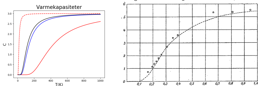
Figur 7.5: Einsteins modell for varmekapasiteter, for stoffer med forskjellig karakteristisk temperatur, altså forskjellig fjærkonstant i vibrasjonene (til venstre). Denne modellen var publisert i 1907. Figuren til høyre er tatt fra Einsteins publikasjon og viser modellen sammelignet med datapunkter for diamant.
