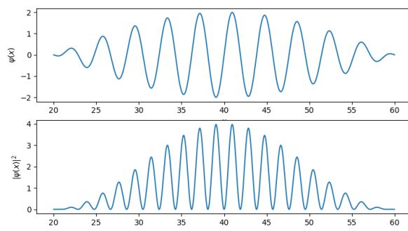
Figur 3.3: Bølgepakke satt sammen av to litt ulike frekvenser, f_0 = \nu_0 = 0,25 og f_1 = \nu_0 + 0,1 \times \nu_0 . Amplitude og intensitet på et gitt tidspunkt som funksjon av posisjon. Man får en omhyllingskurve med frekvens lik \nu_1 - \nu_0 . I kvantemekanikken tolkes |\psi(x)|^2 dx som sannsynlighet for å finne partikkelen mellom posisjon x og x + d(x)
