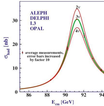
Figur 10.16: Målt virkningstverrsnitt for prosessen e^+e^- \rightarrow q\bar{q} i energiområdet rundt m_{Z^0}c^2 , sammenlignet med teoretisk forutsigelse for forskjellig antall nøytrinofamilier.
