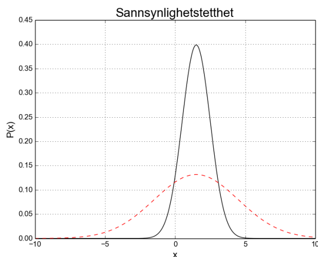
Figur 3.1: Eksempel på sannsynlighetstetthetsfunksjoner, P(x) = \psi^* \psi , for å finne partikkel i posisjon x . Kurvene viser gaussfordelinger med størst sannsynlighet i x = 1, 5 , men med forskjellig standardavvik, h.h.v \sigma = 1 (heltrukket), og \sigma = 3 (stiplet).
