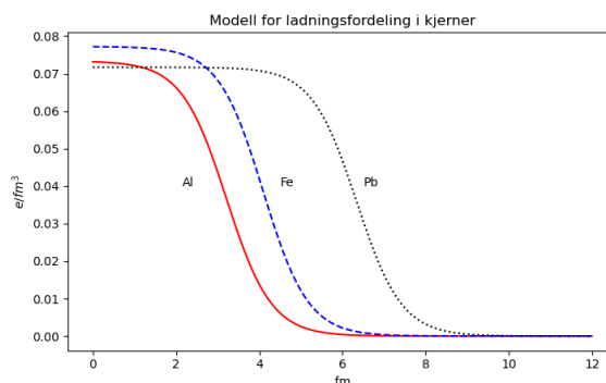
Figur 9.2: Modell av elektrisk ladningsfordeling i kjerner
