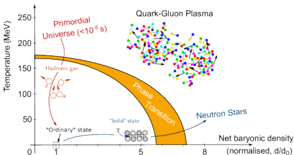
Figur 11.5: Fasediagram for hadonmaterie. I det tidlige univers var det svært høy temperatur, og materien eksisterte som et plasma. Dette er et sted høyt oppe på y-aksen. I tungionekollisjoner skaper man plasmaet ved å lage systemer med svært høy tetthet. (Fra CERN, ALICE-PHO-SKE-2015-002)
