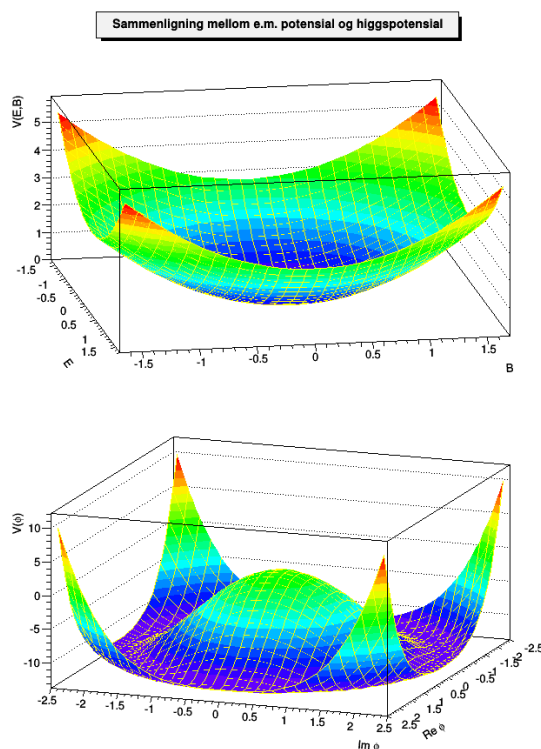
Figur 10.18: Det elektromagnetiske potensial (øverst) og Higgspotensialet (nederst) som funksjon av sine respektive felter (enheter på aksene er helt vilkårlige)
