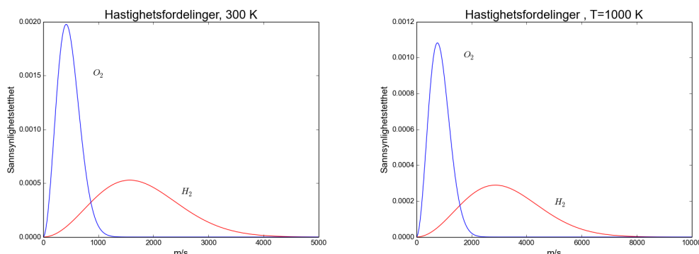
Figur 7.2: Maxwell-Boltzmanns hastighetsfordelinger for to gasser og temperaturer (Legg merke til at aksene er forskjellige i de to plottene.
