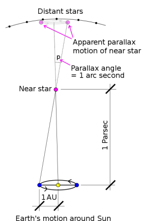
Figur 11.1: Definisjon av lengdeenheten Parsec. Fra Wikipedia. Stjernen 'Near star' ser ut til å ha flyttet på seg fra den ble observert i desember til den ble observert i juni. Posisjon er observert relativt til en bakgrunn av andre stjerner som ligger så langt borte at de observeres som stillestående. Forskjell i vinkel som retningen til stjernen danner med bakgrunnen gir informasjon om avstanden til stjernen. Om stjernen tilsynelatende har flyttet mye på seg så ligger den nærmere enn når den tilsynelatende har flyttet lite på seg. Siden vi kjenner radien til solbanen og måler 'Parallakse-vinkelen', så kan vi beregne avstanden til stjernen.
