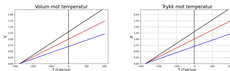
Figur 7.1: Stiliserte sammenhenger mellom temperatur for gassvolum ved konstant trykk og gasstrykk ved konstant volum
