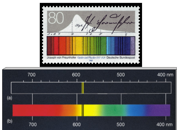
Figur 5.4: Lys fra sola med absorpsjonsspektrum som kolorert av Fraunhofer selv. Fra Wikipedia. Nederst: Na-absorpsjonsspektra, og emisjonsspektra. Fra https://chemistry.stackexchange.com/
