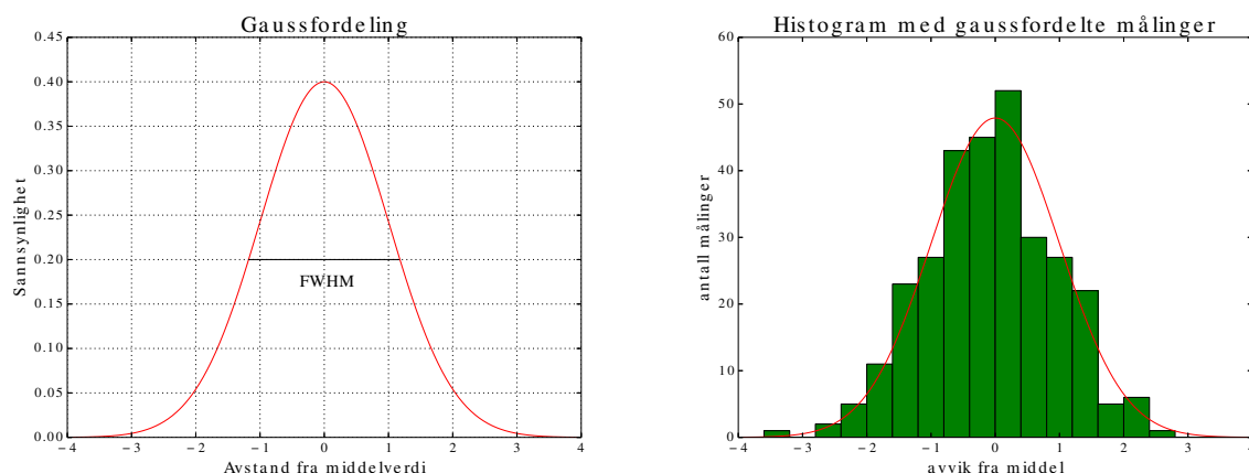
Figur B.1: a) Gaussfordeling med middelværdi 0 og standardavvik 1, b) Histogram med 300 tilfeldig genererte måleresultat som følger denne sannsynlighetsfunksjonen
