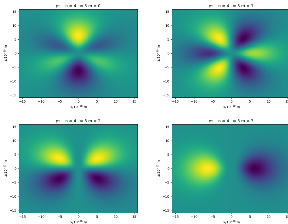
Figur 4.6: Funksjonsverdier for de fire bølgefunksjonene med n = 4 og l = 3 i z - x planet. Realdelen av funksjonen er plottet (i dette planet er imaginærdelen lik 0, siden vi har \phi = 0 for positiv x , og \phi = \pi for negativ x ). De mørkeblå partiene har lavest funksjonsverdi, med \psi < 0 . De lysegule partiene har høyest funksjonsverdi og \psi > 0 . Det er 'automatisk' fargeskala. Enheter på aksene er i Ångstrøm. Legg også merke til at alle funksjonene er odde når koordinatene skifter fortegn, x \rightarrow -x og z \rightarrow -z (og y \rightarrow -y ). De har paritet lik -1, i tråd med forventning, som er at pariteten til bølgefunksjonene er gitt som (-1)^l .
