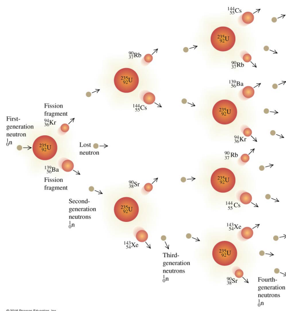
Figur 9.19: Kjedereaksjon (Fra [17])
