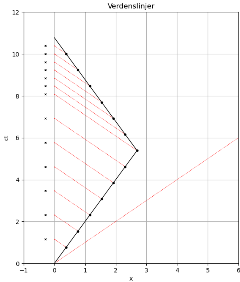
Figur 1.3: En verdenslinje i tidrommet for et objekt med hastighet \beta = 0,5 , og linjer for lyssignaler som sendes 'hjem' med jevne mellomrom. Kryssene til venstre viser tidspunkt for mottak av signalene som beregnet med formel 1.8. Linja for lyssignal, ct = x er også vist
