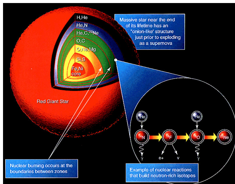
Figur 9.25: Figuren viser hvor de tyngre grunnstoffene er laget i tyngre stjerner (fra Wikipedia)
