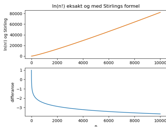
Figur 7.4: Stirlings formel for tilnærming av \ln n! . Det øverste panelet viser den eksakte formelen og tilnærmingen. Siden den relative forskjellen er så liten, er det ikke mulig å skjelne de to kurvene fra hverandre. Den nederste figuren viser forskjellen mellom de to kurvene. Vi har altså en relativ feil i Stirlings formel på omtrent 3/80000 når n = 10000 .
