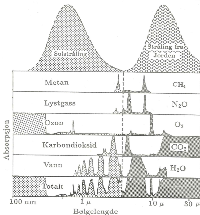
Figur 6.3: Strålingsspektre fra sola og jorda, og absorpsjonsspektra for noen av de viktigste atmosfæregassene. Vi ser at det er klar separasjon mellom strålingsspektrene til den varme sola og den mye kaldere jorda. Absorpsjonsspektrene til de forskjellige gassene er skravert forskjellig i to områder, for å vise om det er hovedsakelig solstråling eller jordstråling som absorberes (fra [10]).
