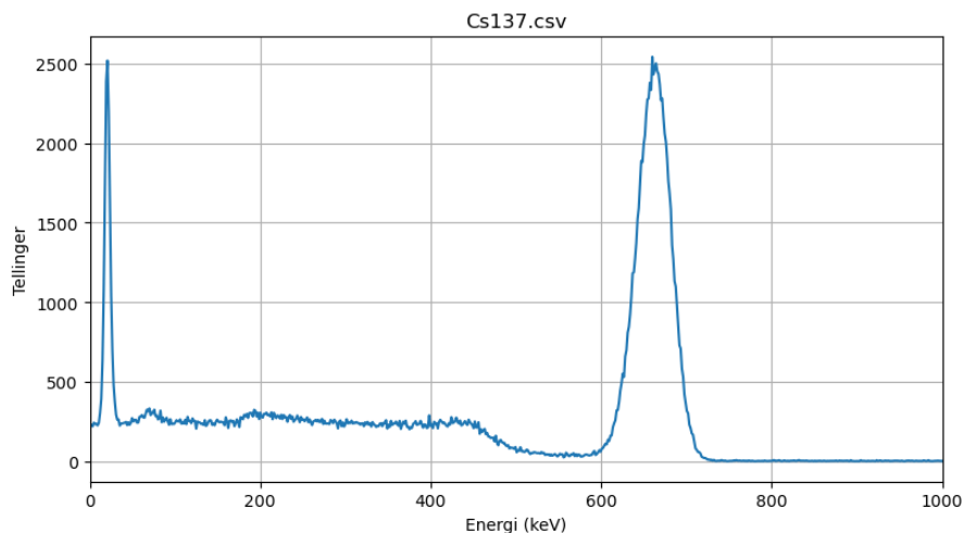
Figur 2.5: Spektrum av ioniseringer når høyeenergetiske fotoner treffer et materiale. Mange av prosessene som fotoner har i vekselvirkning med materie kan oppsummeres i denne figuren. Fotonene selv lager ikke signaler, de må først vekselvirke i skyen av elektroner i materialet; overføre hele, eller deler av sin energi til ett elektron, som i sin tur lager ionisasjonsenergi som kan observeres. Figuren viser energiavsetningen fra slike elektroner i et krystall når høyeenergetiske fotoner på 662 keV treffer materialet. Mange fotoner med denne energien har truffet materialet, og plottet viser fordeling av antall fotoner som funksjon av energiavsetning. Den fotoelektriske effekt forårsaker at all energien overføres til materialet og ses som en topp ved 662 keV. Toppens bredde skyldes apparaturens oppløsningsvne. Det er unøyaktighet i energimålingen som gir en spredning i utfall av energimålingen. Den relativt flate fordelingen av energier kommer av Comptonspredning med et spekter av spredningsvinkler fra 0 til 180 grader. Ved 180 grader spredning går altså fotonet tilbake der det kom fra, og energieoverføringen til elektronet er maksimal, ca 475 keV (se ligning 1.21). Den skarpe toppen til venstre skyldes røntgenstråling som har oppstått i forbindelse med den radioaktive prosessen som genererer strålingen. Materialene brukt til å innkapsle den radioaktive kilden kan være bestemmende for nøyaktig posisjon av denne toppen, og hvor mange topper det er.
