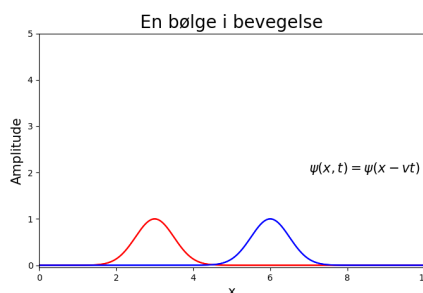
Figur 3.2: En bølgefunksjon som propagerer langs positiv x-akse med tiden. Funksjonen vises ved to forskjellige tidspunkt. Den forskyver seg med tiden, men endrer ikke form.
