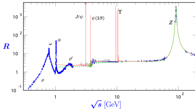
Figur 10.12: Forholdet R (ligning 10.12). De røde 'strekene' er veldig smale og høye resonanser i virkningstverrsnittet. Fra [31]
