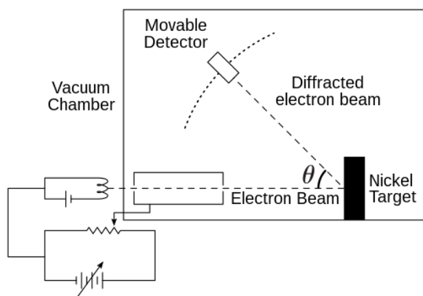
Figur 2.12: Davisson Germer eksperiment. Fra Wikipedia [33]
