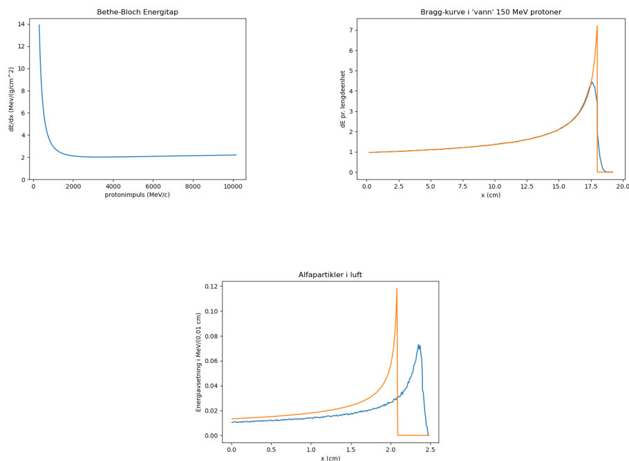
Figur 9.12: Øverst venstre: Spesifikk energiavsetning for protoner som funksjon av protonets bevegelsesmengde. Denne formelen kalles Bethe-Bloch-formelen.
