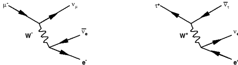
Figur 10.10: Feynman-diagram av: a) \mu^- henfall b) \tau^+ henfall. Verteksfaktorene er her ikke \sqrt{\alpha} , men den svake koblingskonstanten g_W .
