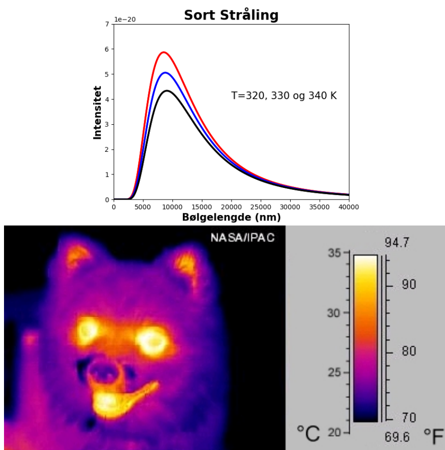
Figur 7.11: Strålingsintensitet varierer sterkt med temperaturen til objektet som stråler. Nederst er et nattbilde med kamera som er følsomt for infrarødt lys. Strålingsintensitet er gjort om til passende farger. Fra Wikipedia.[37]
