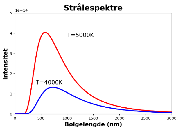
Figur 7.10: Plancks strålingslov for forskjellige temperaturer. Siden total intensitet er proporsjonal med T^4 så blir høydene og arealet under kurvene svært forskjellig.
