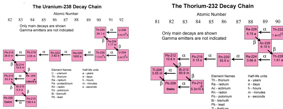
Figur 9.6: Naturlige henfallskjeder.
