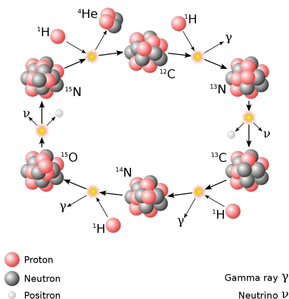
Figur 9.24: Karbon-nitrogen-oksygen prosessen. (fra Wikipedia [50])
