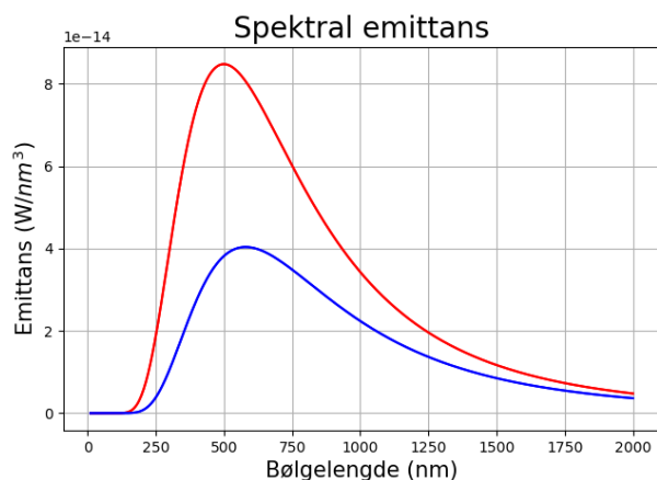
Figur 2.2: Plancks fordelingslov for to temperaturer, 5000K og 5800K. Legg merke til at den utstrålte effekten ved 5800K er mye større enn ved 5000K. Solas overflate har en temperatur på ca 5780 grader.
