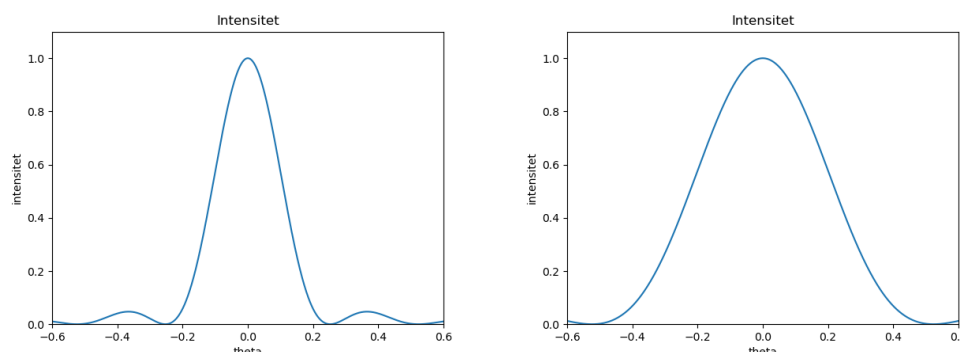
Figur 2.6: Diffraksjonsmønster for lys gjennom en spalte med åpninger på h.h.v. L = 4\lambda og L = 2\lambda . Om vi projiserer strålen på en plate bak spalten så vil intensitetsfordelingen være svært forskjellig fra en firkantet boks bak spalten, slik det hadde vært uten diffraksjon. De gjennomsnittlige retningsendringene for fotoner innenfor første intensitetsminimum er numerisk beregnet til henholdsvis s_\theta = \sqrt{\theta^2} = 0,084 og 0,172 .
