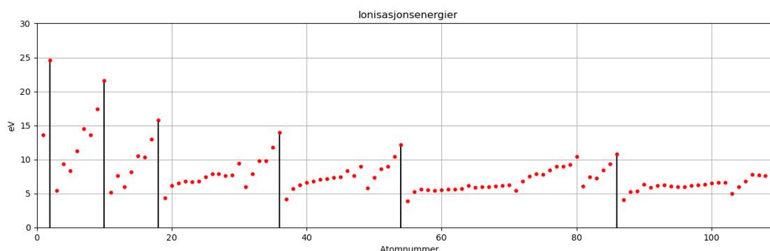
Figur 5.2: Ionisasjonsenergier for elementene. De svarte linjene markerer edelgassene (slutten på en periode). Data fra NIST Atomic Spectra Database, Kramida, A., Ralchenko, Yu., Reader, J., and NIST ASD Team (2023).
